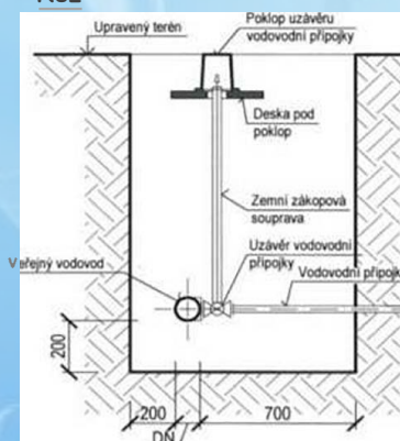
Řez
